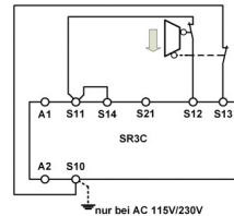
Abb. 7: Zweikanalige Schiebeschützgitter-Überwachung mit Querschluss- und Masseschluss-Überwachung (Kategorie 4, bis PL e / SIL 3)
