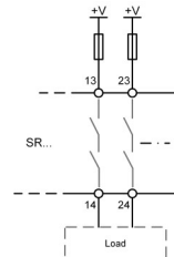
Abb. 15: Anschluss zu schaltender Lasten an Sicherheitskontakte. (Beispielhafte Kontaktanordnung. Je nach Gerätetyp abweichend. Schaltspannungen „+V“ entsprechend techn. Daten)
