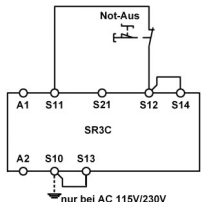
Abb. 6: Einkanalige Not-Halt-Schaltung mit Masseschluss-Überwachung (Kategorie 1, bis PL c / SIL 1)
