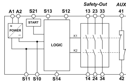
Abb. 1 Blockschaltbild SR3C
