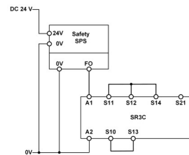
Abb. 9: Anschluss an fehlersichere Steuerung (Kat. 4, bis PL e / SIL 3) Voraussetzung: Fehlerrückmeldung für Querschluss (z.B. gemäß EN ISO 13849-2; Tabelle D4 - Verdrahtung in geschütztem Verdrahtungsraum) und Steuerung erfüllt ebenfalls Anforderungen an Kat. 4, PL e / SIL 3
