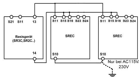
Abb. 6: Rückführkreis
