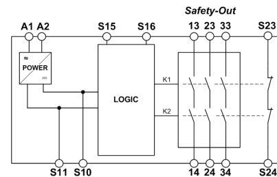
Abb. 1 Blockschaltbild SREC
