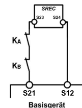
Abb. 7: Rückführkreis mit Auto-Start
