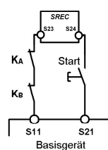
Abb. 6: Rückführkreis
